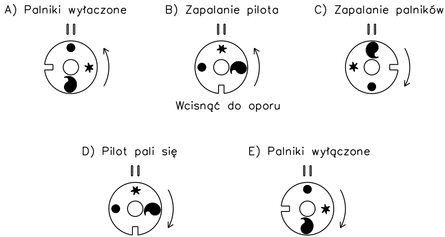
Rysunek 4 - Działanie elektromagnetycznego zaworu gazowego SIT 820 NOVA (Widok pokrętki zaworu)
