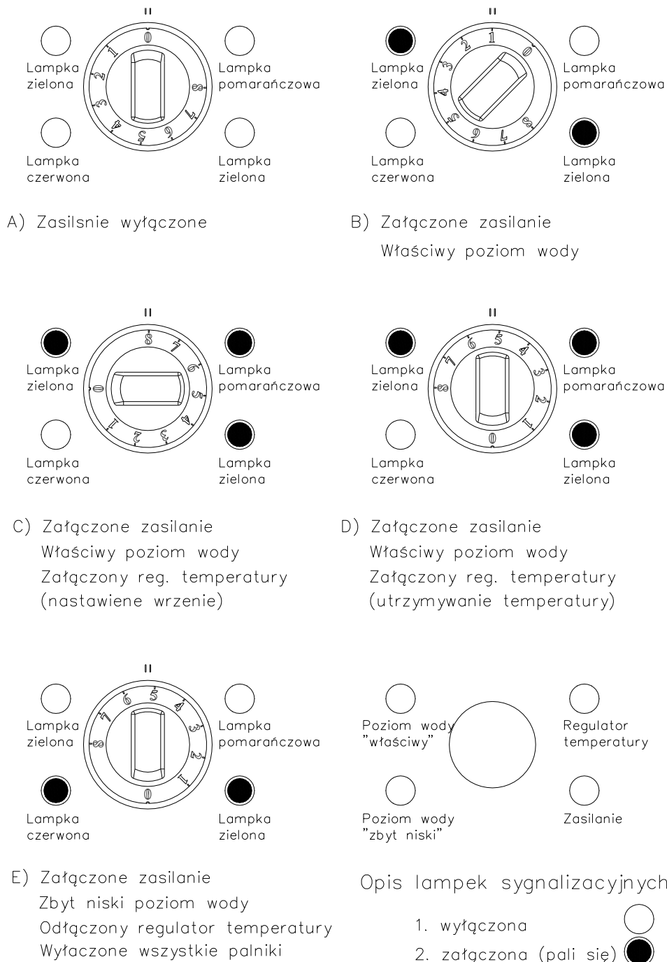
Rysunek 5 - Działanie wyłącznika głównego i regulatora temperatury (Widok pokrętki i sygnalizacji świetlnej)
