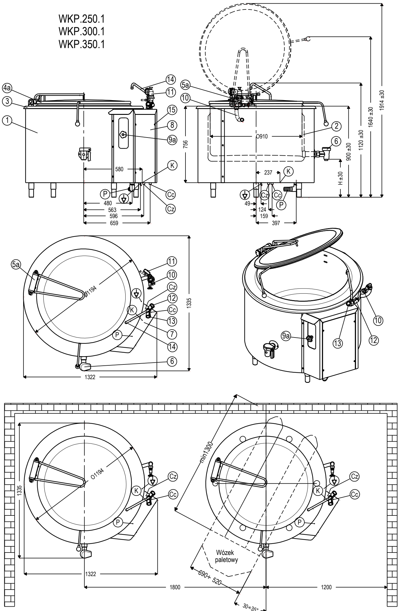
Rysunek.2 – widok ogólny kotłów WKP.250.1, WKP.300.1, WKP.350.1
