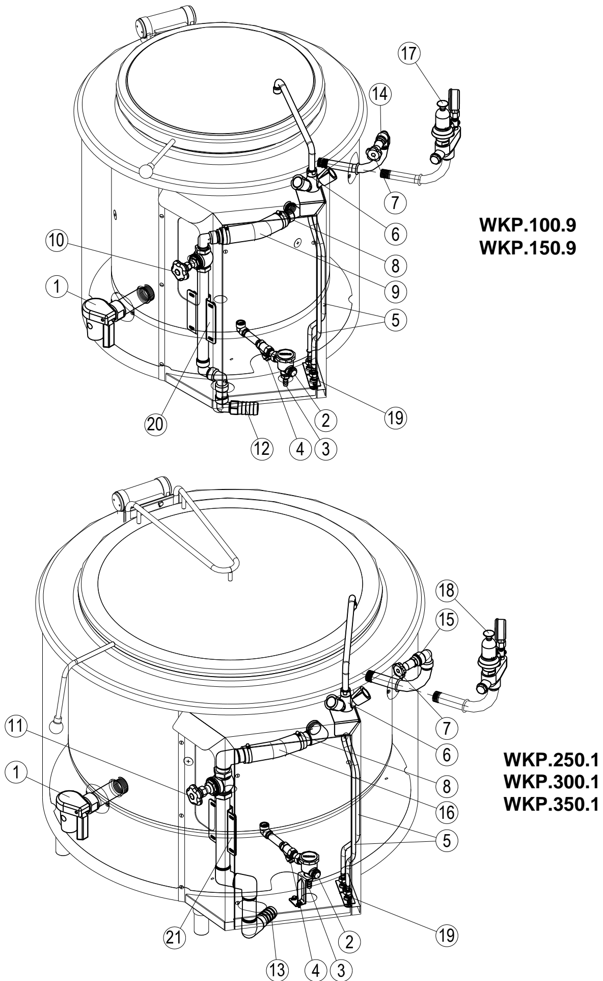
Rysunek 3 – Zespół instalacji kotłów
