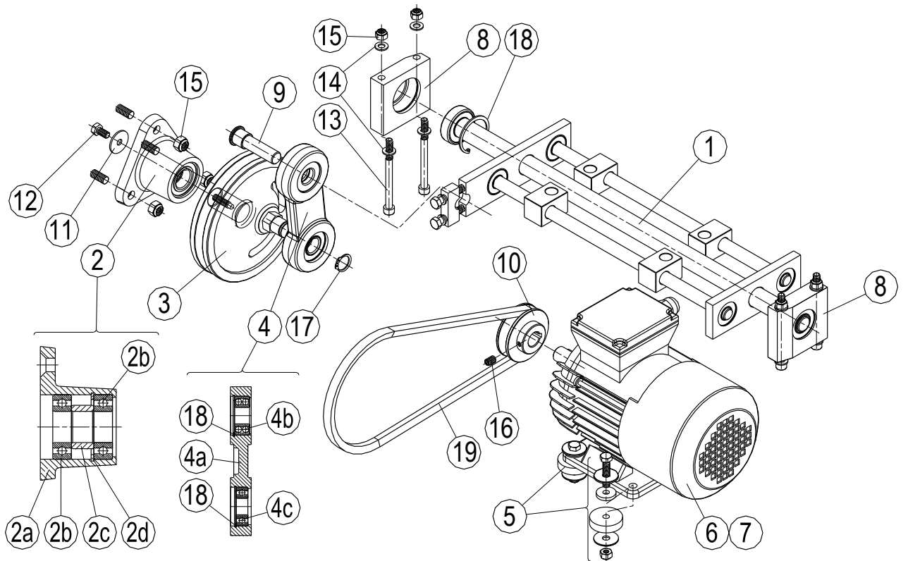
Rysunek 4 - Napęd
